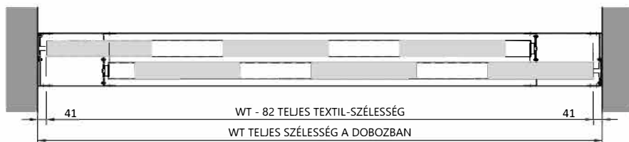
ALAPRAJZ - TÍPUSA: AT-H-E
