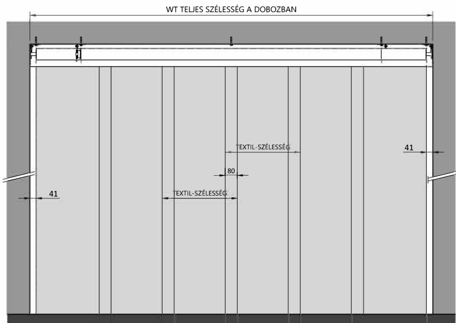
METSZET - TÍPUS: AT-H-E
