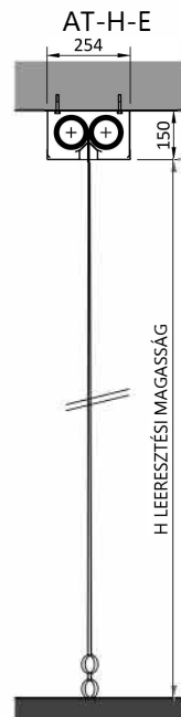
METSZET - TÍPUS: AT-H-E
